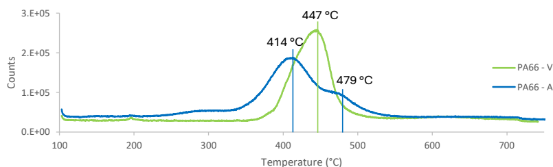
Figura 1. Profili termici di PA-66 vergine (V) e invecchiato (A) ottenuti tramite EGA-MS
