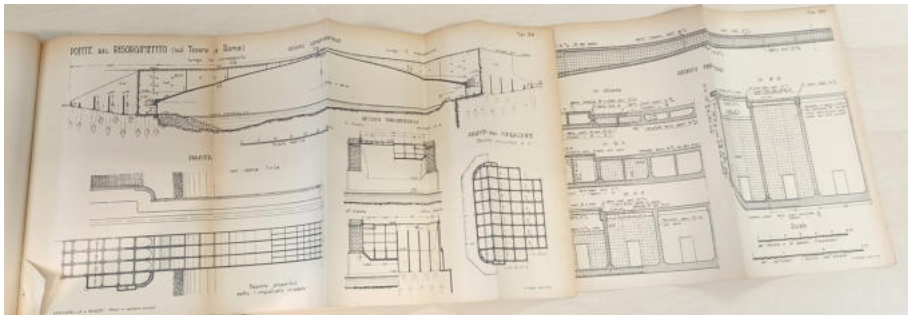
Fig. 22 – L. Santarella e E. Miozzi, Ponti italiani in cemento armato , Hoepli, Milano 1924. Tavole costruttive del Ponte del Risorgimento sul Tevere a Roma.
